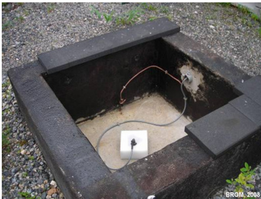
Detall del pou sísmic (acceleròmetre Kinematics Episensor) (fotografia d'estat en construcció, sense coberta)
